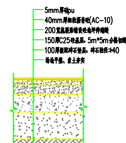
篮球、排球场地构造做法 1 : 1 0
