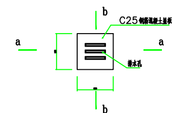
预制钢筋混凝土排水沟盖板 1 : 2 5
