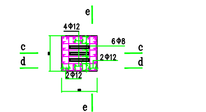
预制钢筋混凝土排水沟盖板配筋 1 : 2 5
