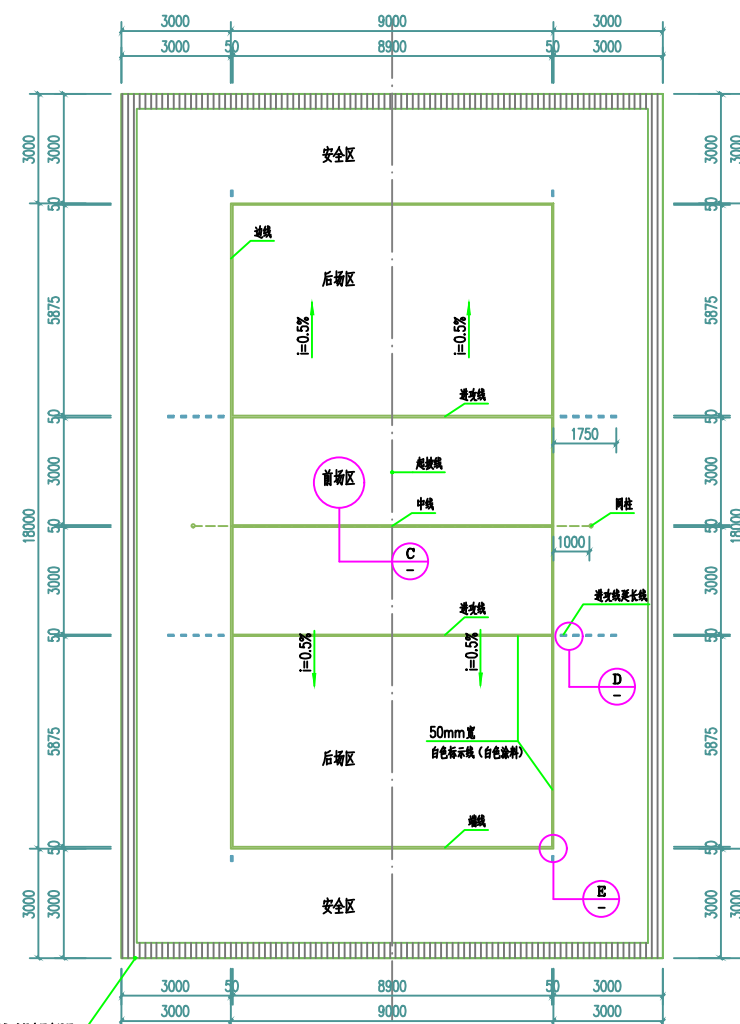
排球平面图 1 : 1 0 0
